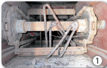
焼却灰搬出装置
